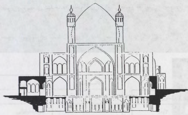
برش ب- ب عرضی و نمای ضلع جنوبی
